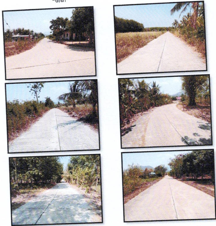
๒. โครงการก่อสร้างถนนคอนกรีตเสริมเหล็ก สายซอยวัง-ชายทะเล ม.๑ ต.ห้วยทราย อ.เมือง จ.ประจวบคีรีขันธ์ งบประมาณ ๑,๙๙๗,๘๐๐ บาท
