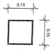
เหล็ก C1 ขนาด 150x150 มม.หนา 3.2 มม.
