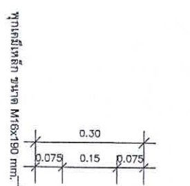
ทุกเหล็ก ขนาด M16x190 มม. แผ่นเหล็ก ขนาด 150x150 มม.หนา 10 มม.
