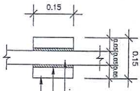
โครงสร้าง T1,T2 แผ่นเหล็ก ขนาด 150x150 มม.หนา 10 มม.
